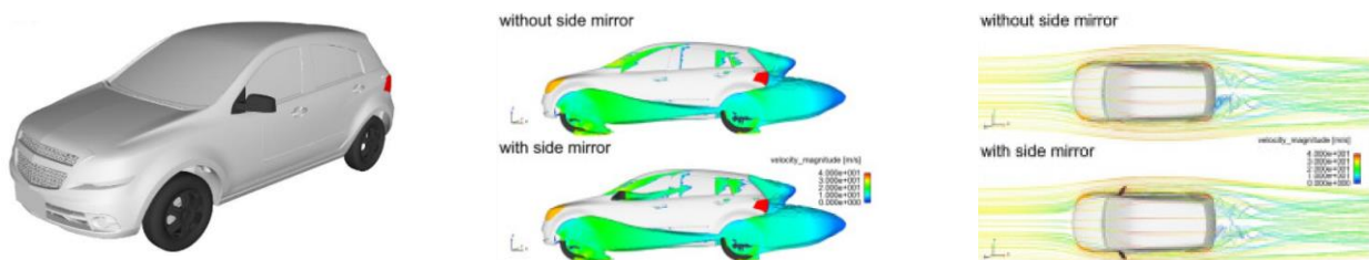
Figura 3. Geometria, contornos de velocidade e linhas de corrente ao redor de um veículo de passeio (Rosilho, 2013)
