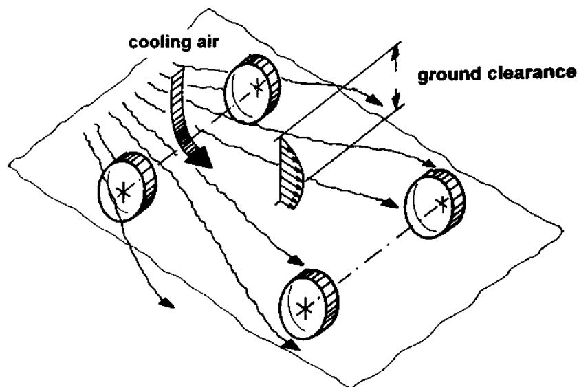
Figura 1. Campo de escoamento na parte inferior do veículo. Ilustração do escoamento de arrefecimento se misturando com o escoamento da parte inferior do veículo (entre o veículo e o chão).
